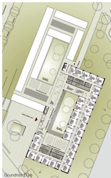
Grundriss EG
